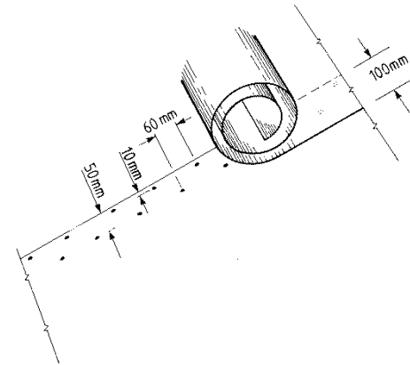
Fig. 7.3.1 "Sikksakkspikring" av asfalt takbelegg eller takfolie
