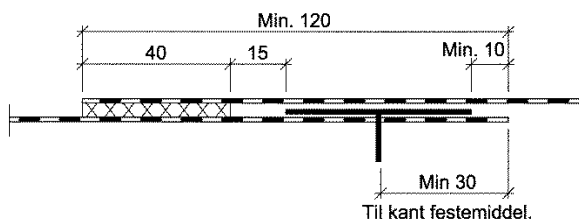
Fig. 5.4.1 Takfolie. Feste i kant av bane
