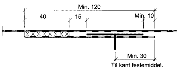
Fig. 5.4.2 Takfolie. Feste i underliggende flipp
