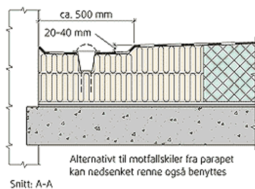
Snitt: A-A
