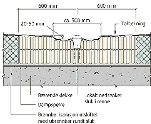
Snitt: A-A
